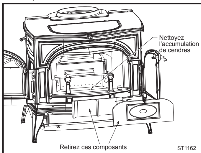
Fig. 47 Inspectez et nettoyez l'accumulation de cendres derrière le système de combustion.
