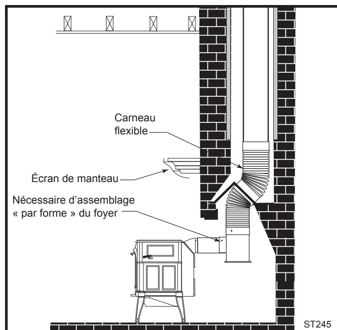
Fig. 9 Installation par de foyer.
