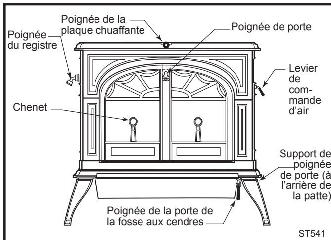
Fig. 31 Les commandes du Defiant sont placées à portée de main et faciles à utiliser.
