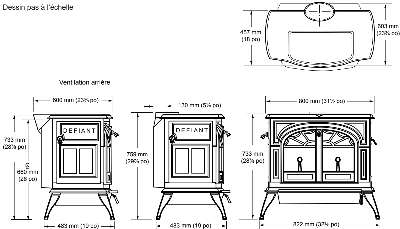
Fig. 1 Dimensions du modèle Defiant.
