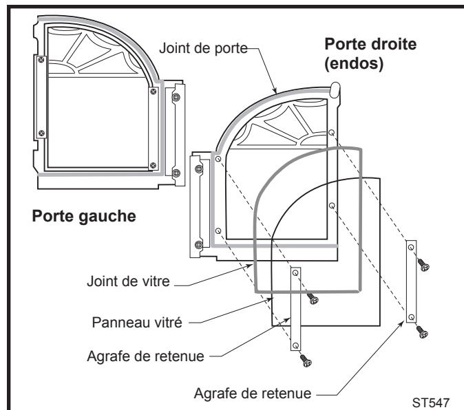
Fig. 42 Vue éclatée de l'ensemble vitré.
