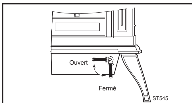
Fig. 40 Tournez la poignée du cendrier dans le sens des aiguilles d'une montre pour l'ouvrir et dans le sens contraire des aiguilles d'une montre pour le fermer.
